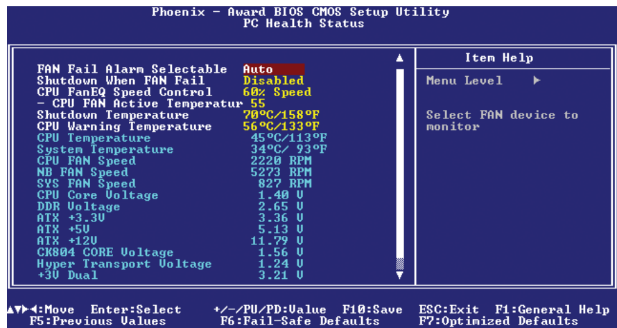
• Figure 10.36 CMOS fan options
