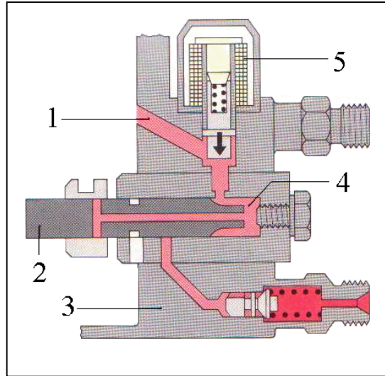
Hình . Van cắt nhiên liệu bằng điện
