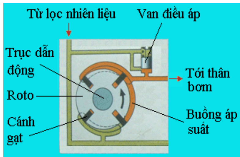
Hình 28. Bơm cánh gạt
