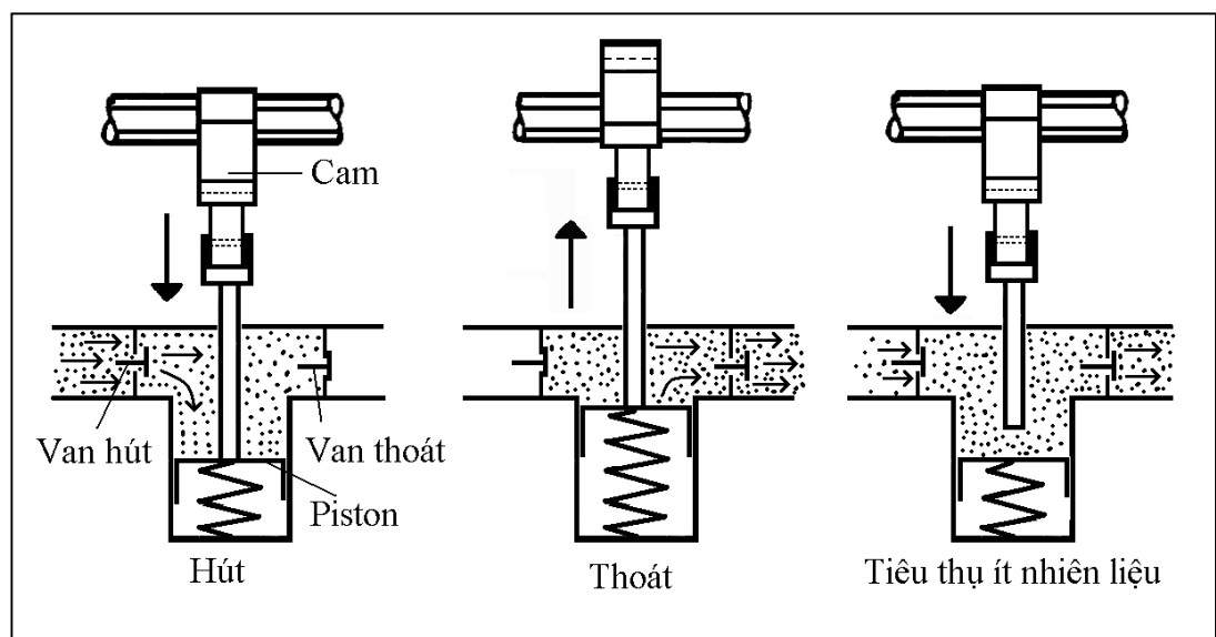
Hình 23. Bơm piston kiểu PM
