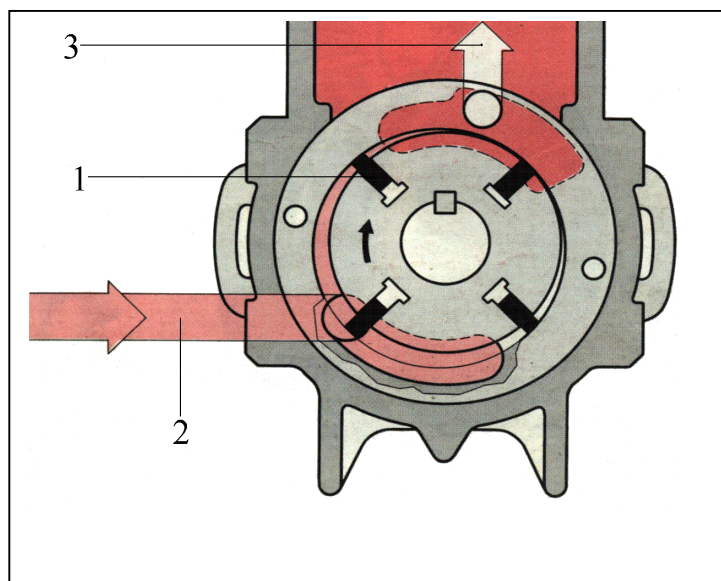
Hình. Bơm cánh gạt
