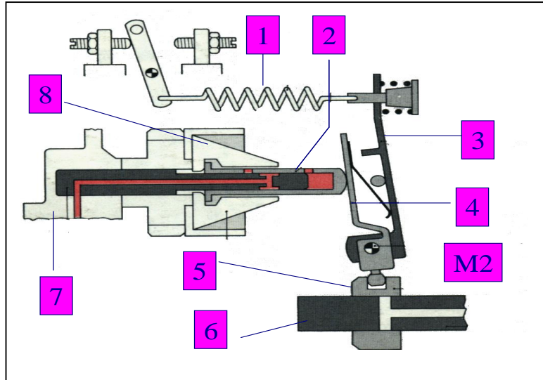
Hình. Bộ Phun Sớm Theo Tải (LFB).
