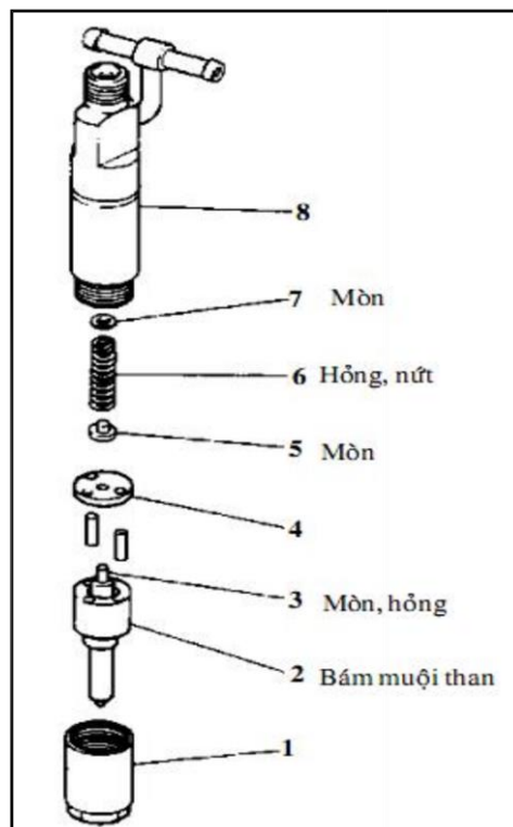
Hình. Trình tự tháo vòi phun loại 1 lò xo.
