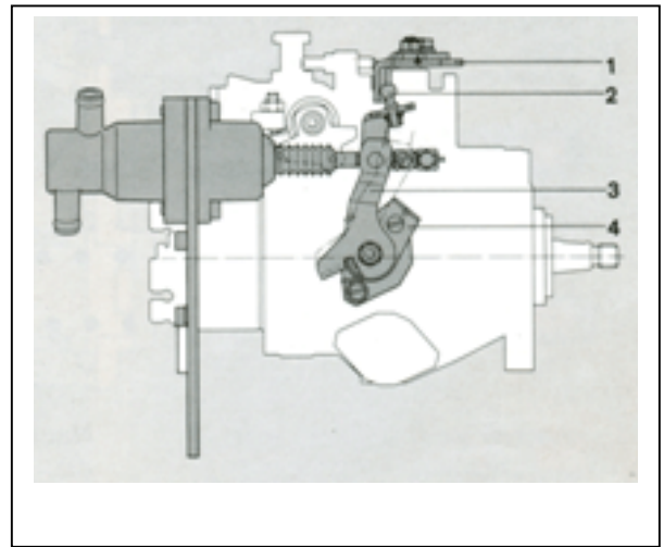
Hình . Bộ cầm chừng nhanh phụ thuộc vào nhiệt độ TLA
