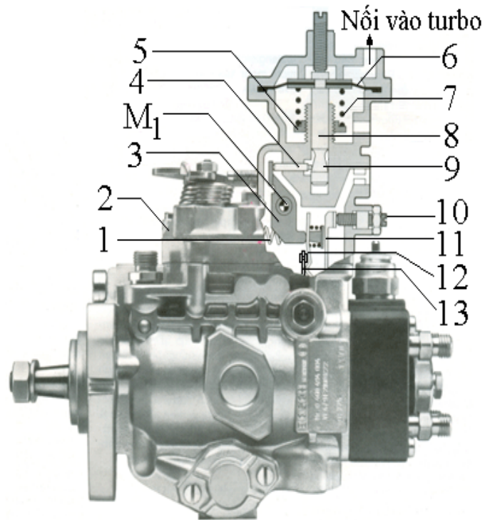
Hình. Cấu tạo bộ bù áp lực
