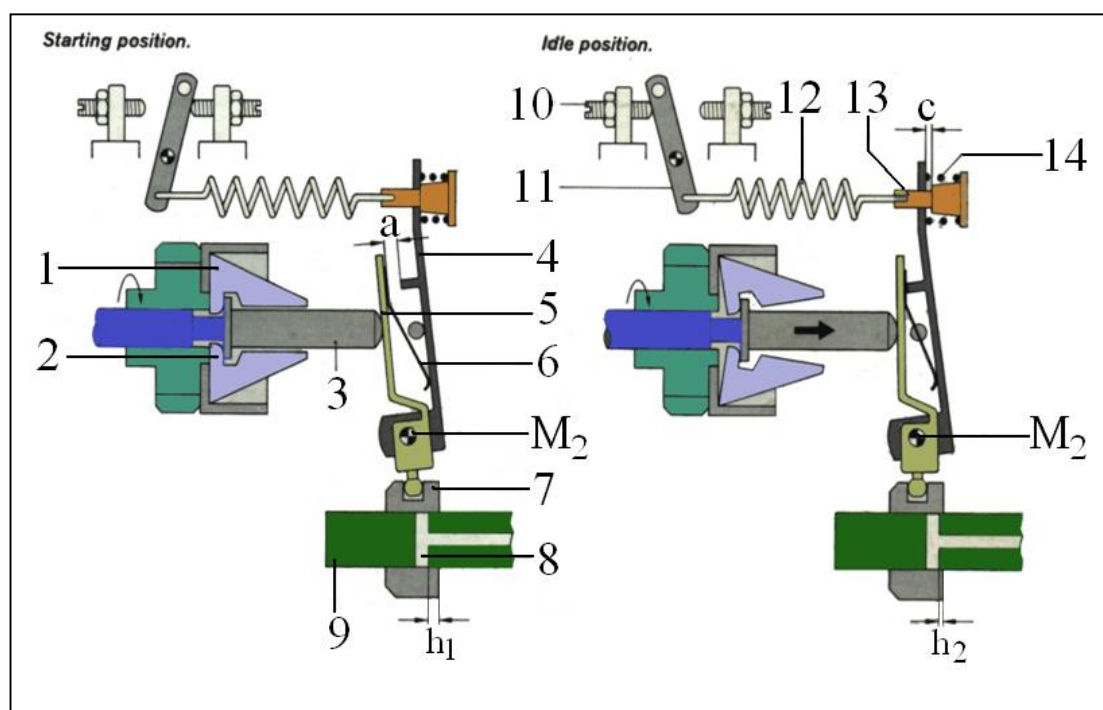
Hình. Bộ điều tốc nhiều chế độ
