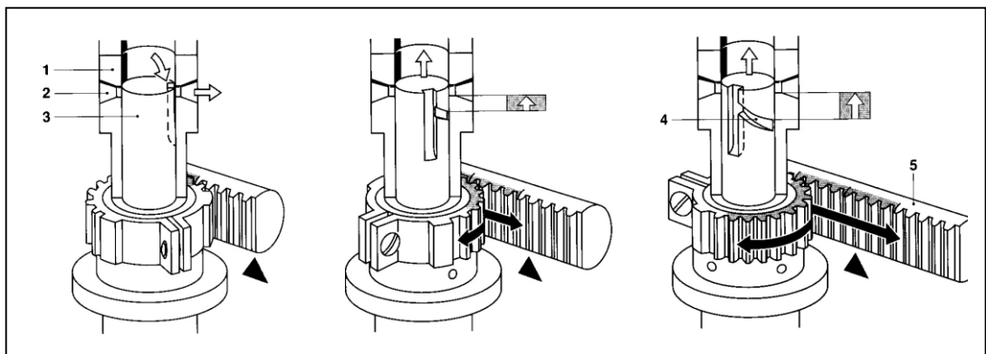
1. Xilanh 2. Lỗ nạp 3. Piston 4. lắn vạt xéo 5. Thanh răng
