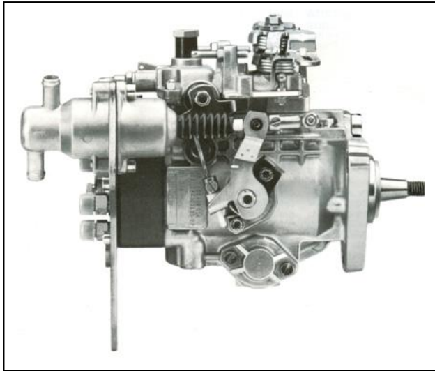
Hình . Bộ cầm chừng nhanh phụ thuộc vào nhiệt độ TLA
