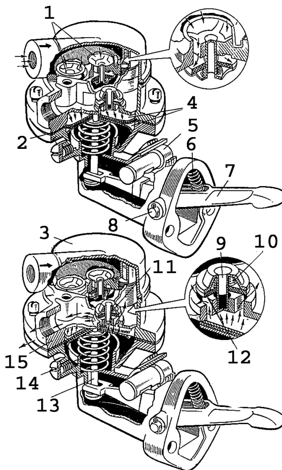
Hình 1.14. Bơm xả cơ khí kiểu màng
