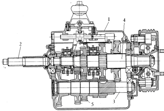
Hình 1.21 Hộp số nằm dọc
