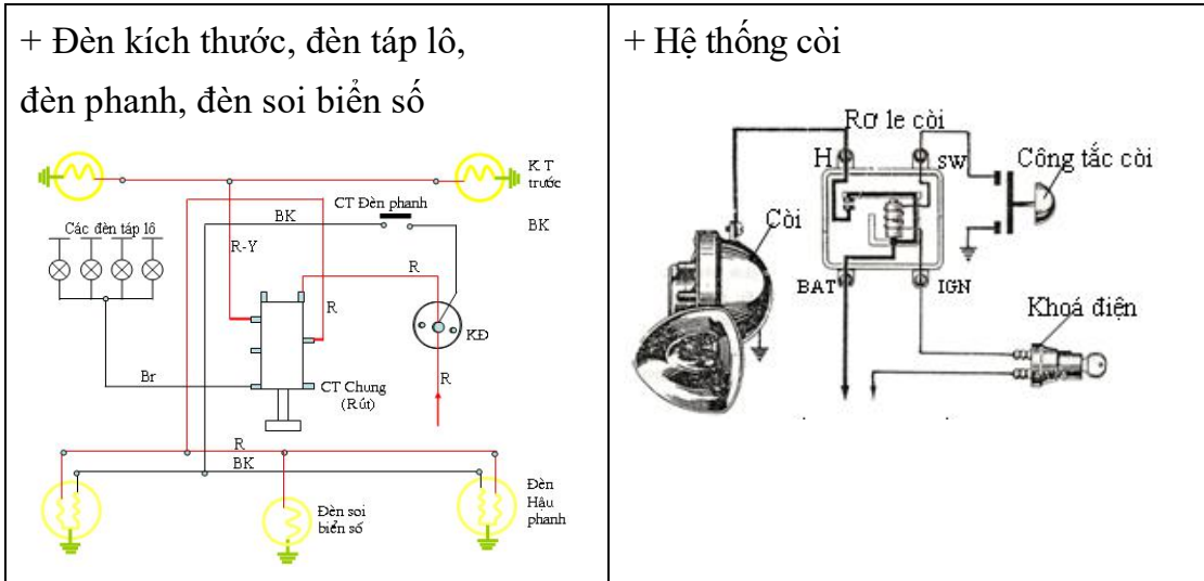
Hình 1.29 : Hệ thống chiếu sáng, tín hiệu
