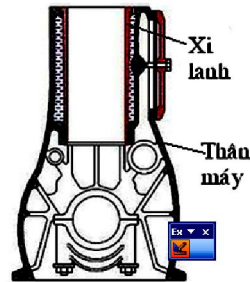
Hình 1.15 Cấu tạo xy lanh trong thân máy
