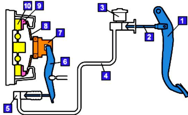
Hình 1.20 Cấu tạo ly hợp
