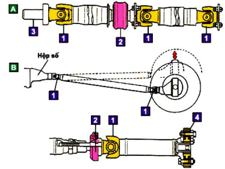
Hình 1.23 cấu tạo các đăng
