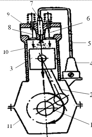
Hình 3.4: Sơ đồ cấu tạo động cơ Diesel
