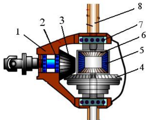
Hình 1.24 Cấu tạo cầu chủ động
