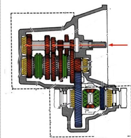
Hình 1.22 Hộp số nằm ngang
