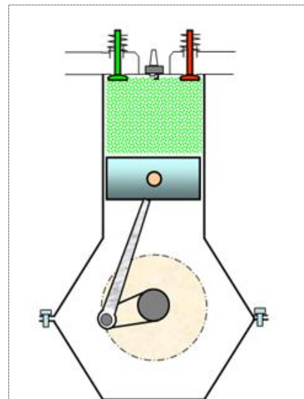
Hình 3.2 b: kỳ ép
