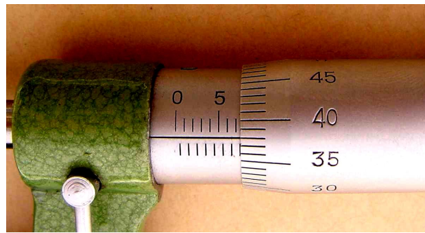
Hình 7.4: Cách đọc trị số trên pan me
