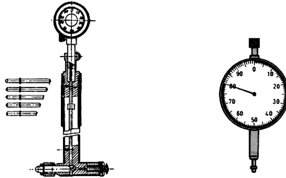
Hình 7.5: Cấu tạo đồng hồ hồ so
