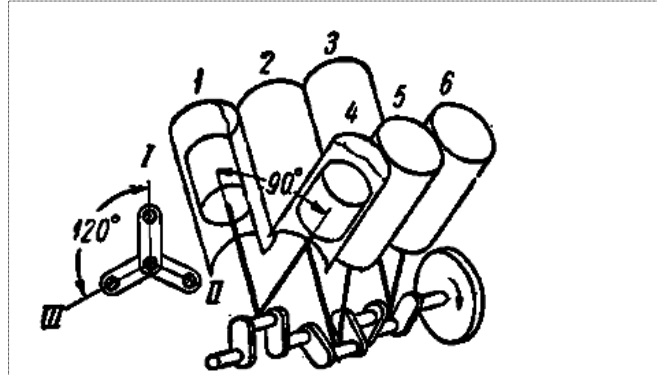
Hình 4.3 Cấu tạo trục khuỷu xếp chữ V
