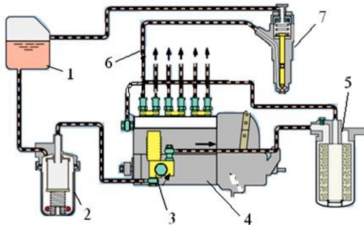
Hình 1.8 Hệ thống cung cấp nhiên liệu Diesel
