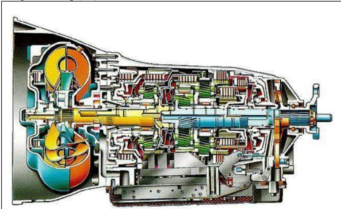
- Hộp số tự động (AT)
