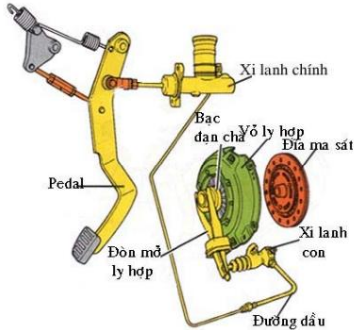
Hình 1.11 Ly hợp dẫn động thủy lực
