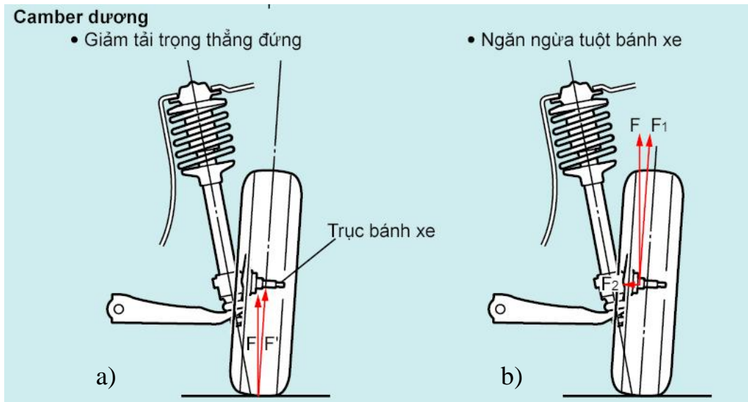
Hình 4.5. Góc camber dương
