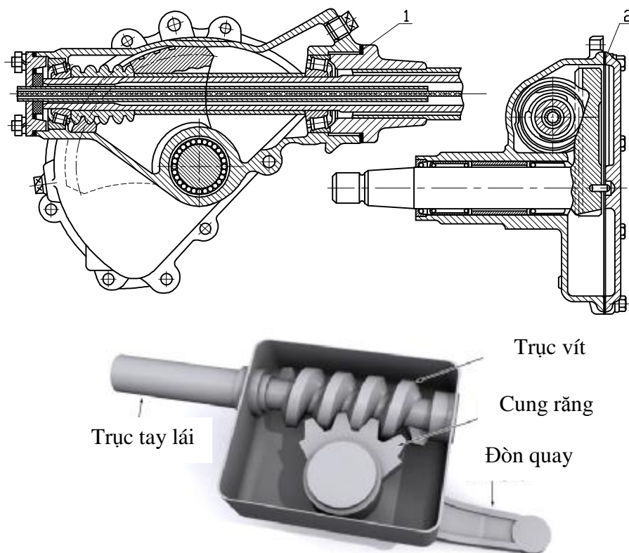
Hình 2.1. Cơ cấu lái trực vít cung răng
