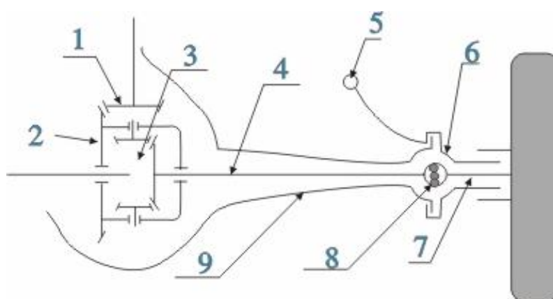
Hình 4.2. Cầu dẫn hướng chủ động
