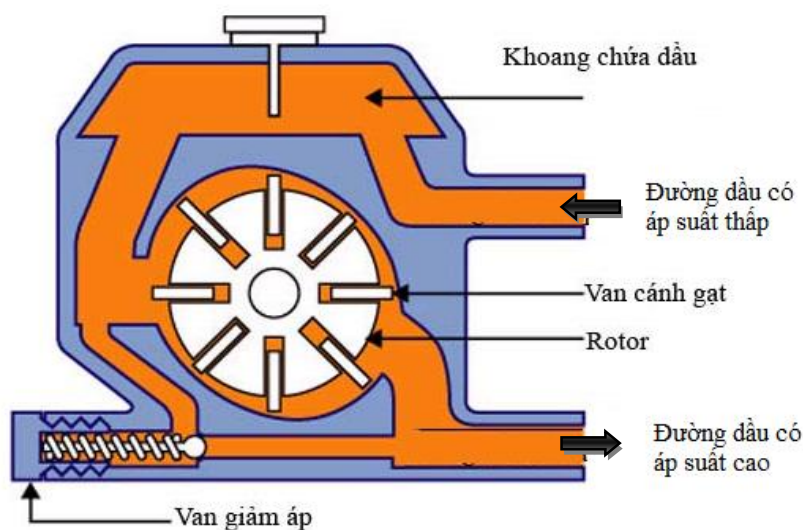
Hình 5.1. Bơm trợ lực lái kiểu cánh gạt
