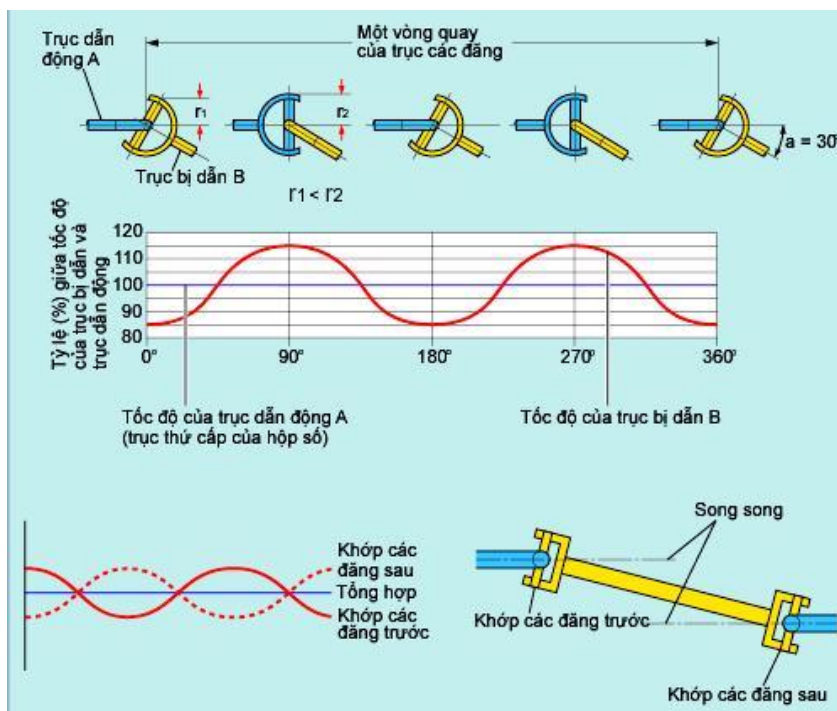
Hình 4.2 Động học của các dạng khác tốc
