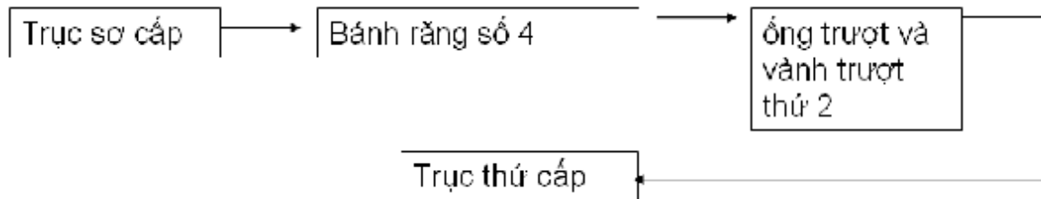
Hình 3.7 Dòng truyền mô men khi gài số 4
