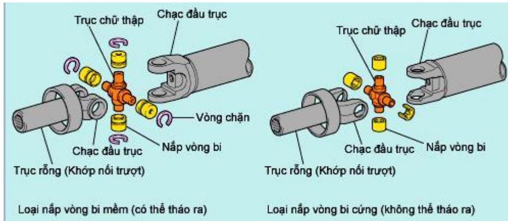
* Động học Hình 4.1 Sơ đồ cấu tạo các dạng khác tốc
