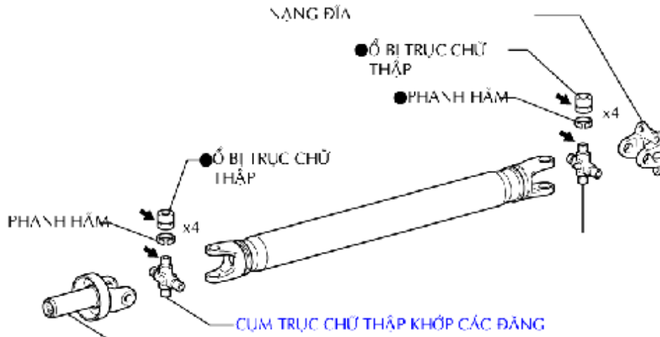
Hình 4.4 Trục các đăng sử dụng hai khớp chữ thập
