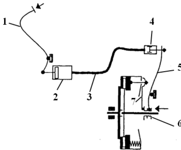
Hình 2.17 Dẫn động thủy lực
