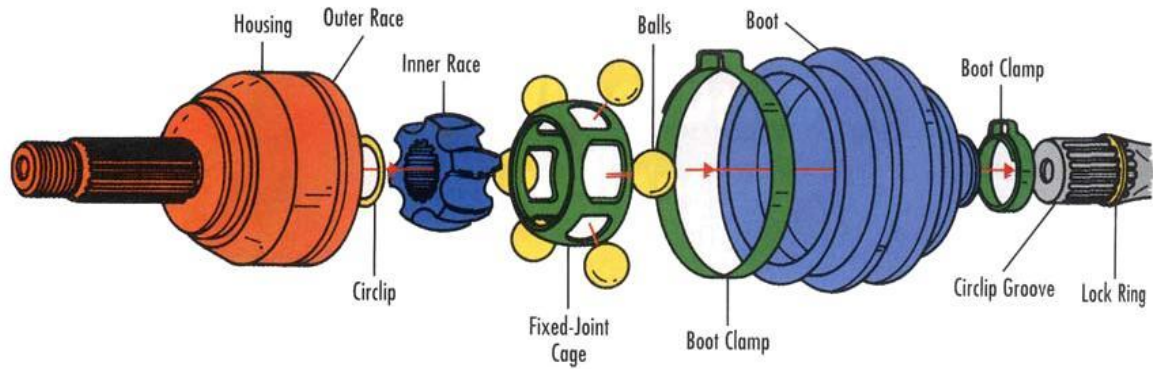
Hình 4.10 Các đăng đồng tốc bi kiểu Rzeppa
